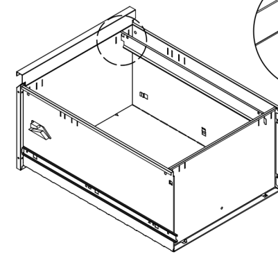
Připevněte závěsné tyče k panelům zásuvek podle obrázku.
