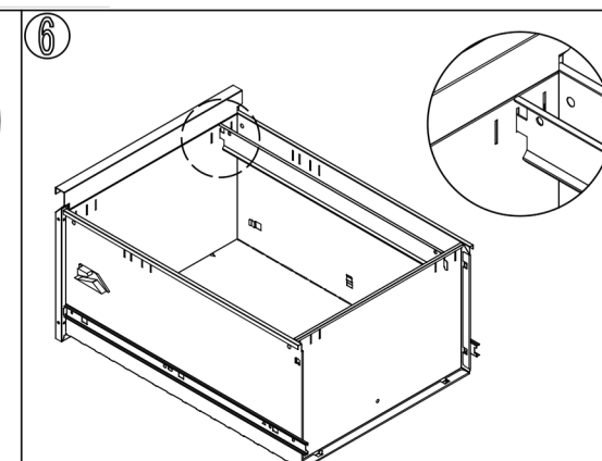
Pritvirtinkite pakabinimo strypus prie stalčių plokščių pagal paveikslėlį.
