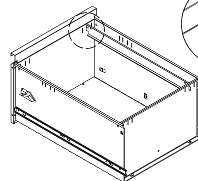
Upevnite závesné tyče k panelom zásuviek podľa obrázka.
